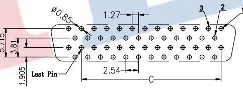
P.C. BOARD LAYOUT (50Pin) R2 Type / 反脚位
