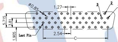
P.C. BOARD LAYOUT (50Pin) R1 Type / 正脚位
